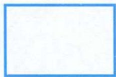
прямоугольник
