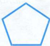
пятиугольник
