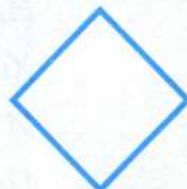
ромб
